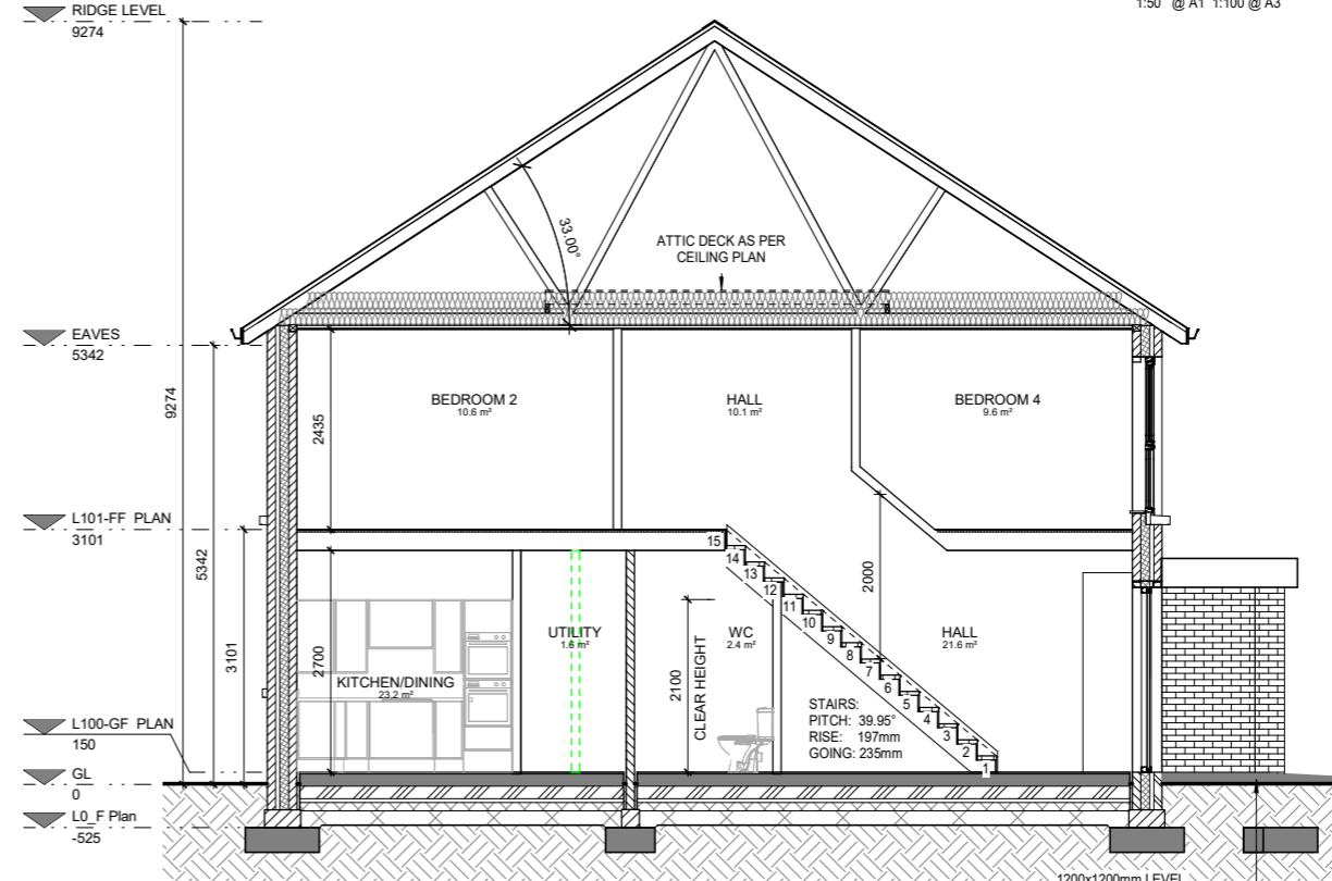
SECTION B-B SEMI 1: 50 @ A1 1:100 @ A3
