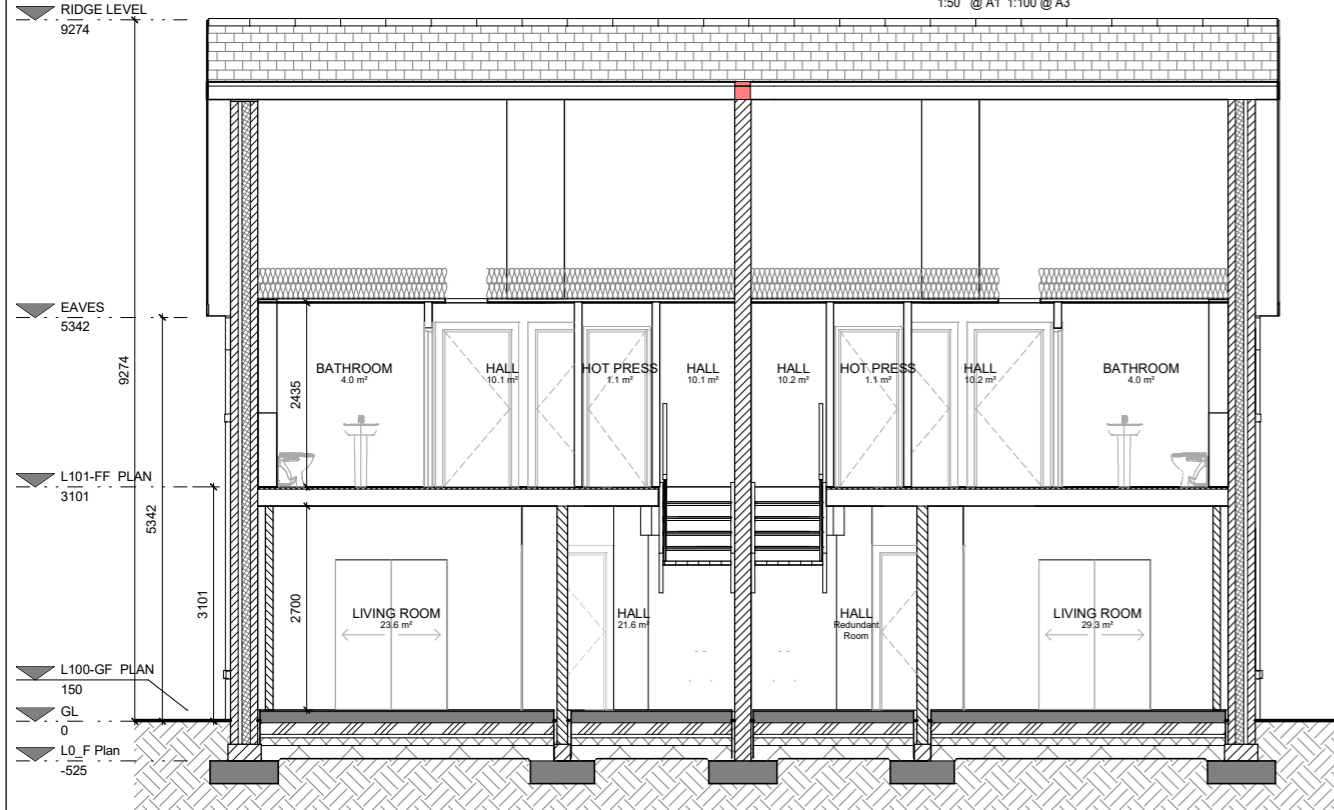
SECTION A-A SEMI 1: 50 @ A1 1:100 @ A3
