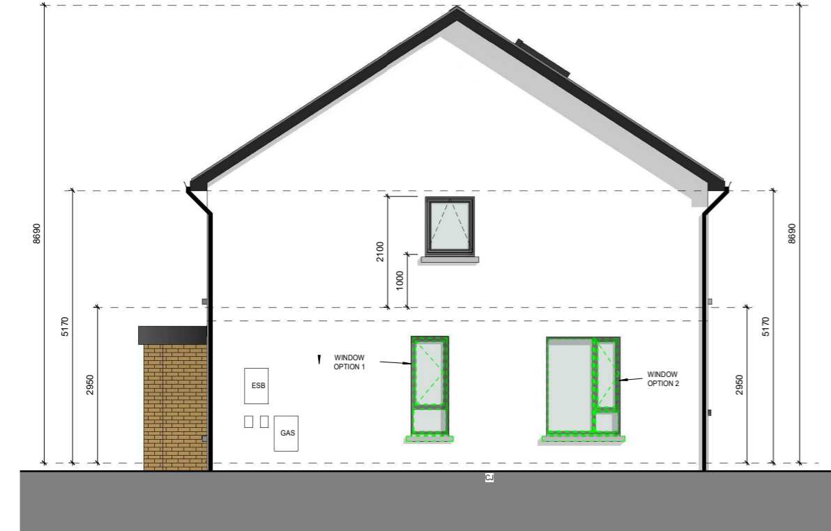
SIDE ELEVATION B 1: 50 @ A1 1:100 @ A3
